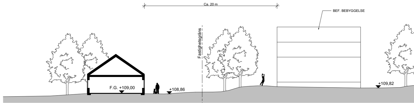
Sektion C-C 1:300
