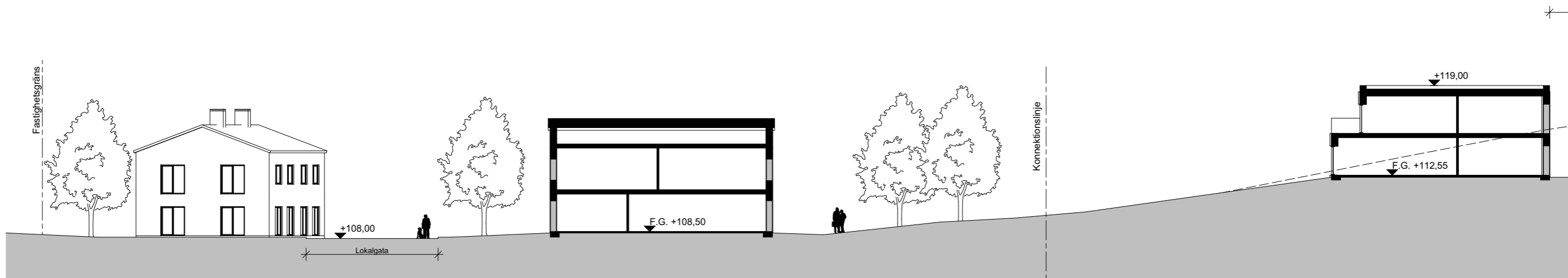
Sektion A-A 1:300
